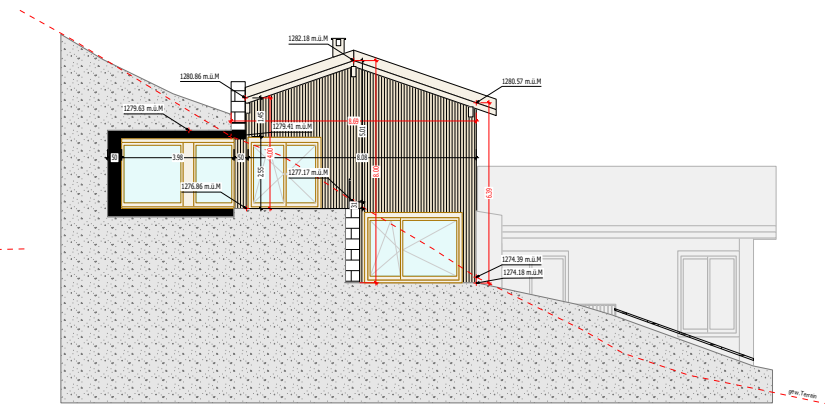
Westfassade
