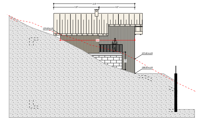
Westfassade
