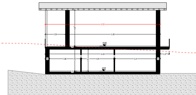
S-02
