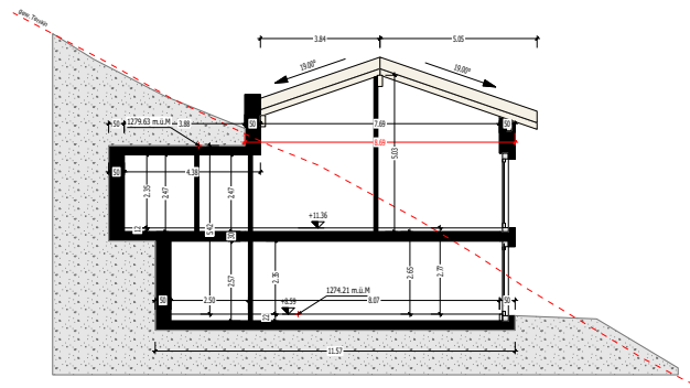
S-01
