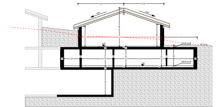
S-02
