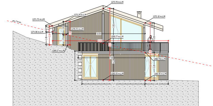
Westfassade
