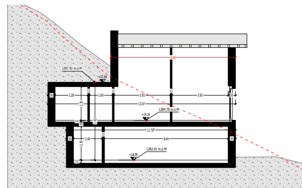
S-01
