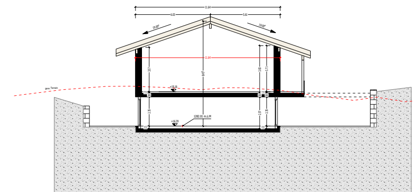
S-02
