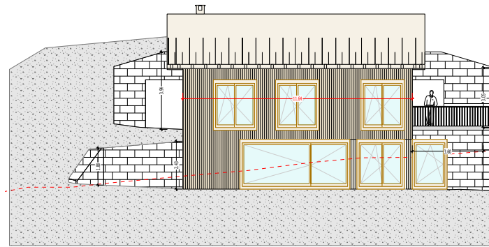
Südfassade
