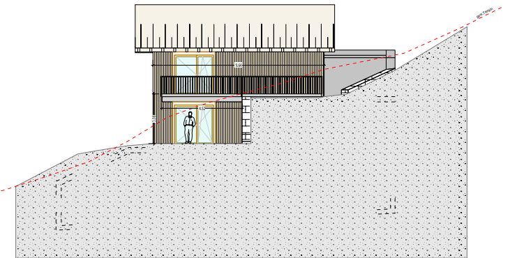
Ostseite
