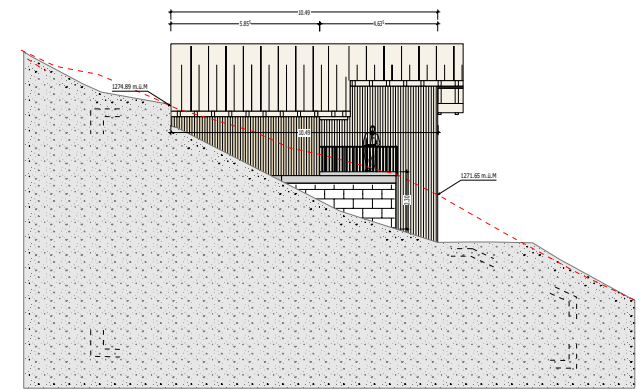
Westseite
