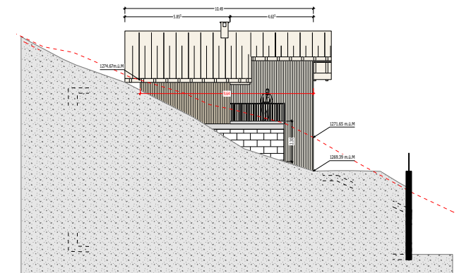
Westseite
