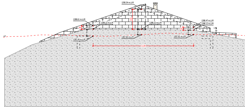
Nordfassade
