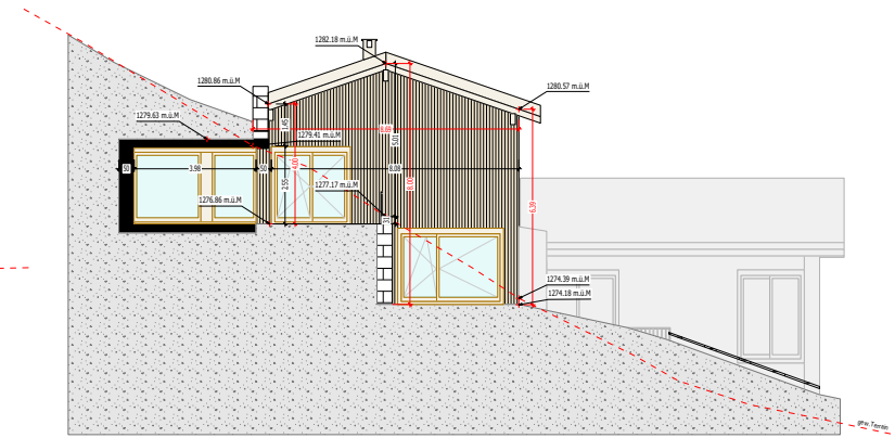
Westseite
