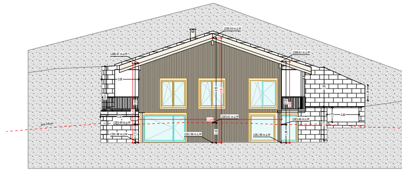
Südfassade
