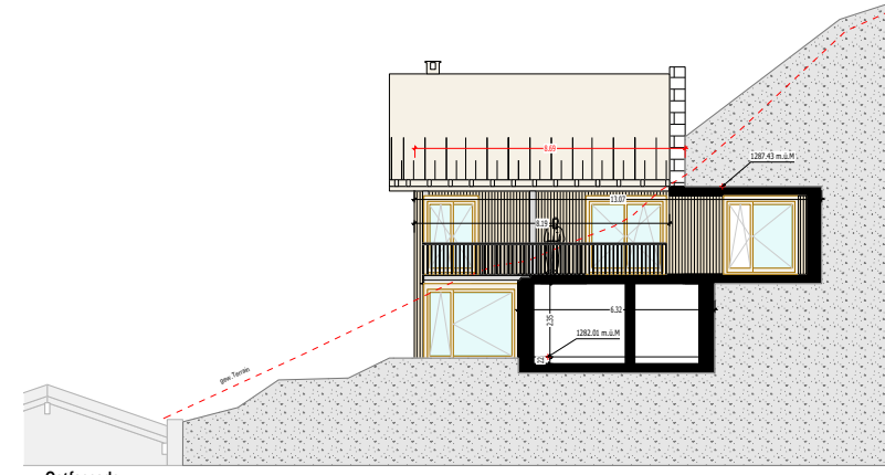
Ostfassade
