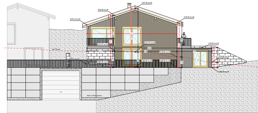
Südseite
