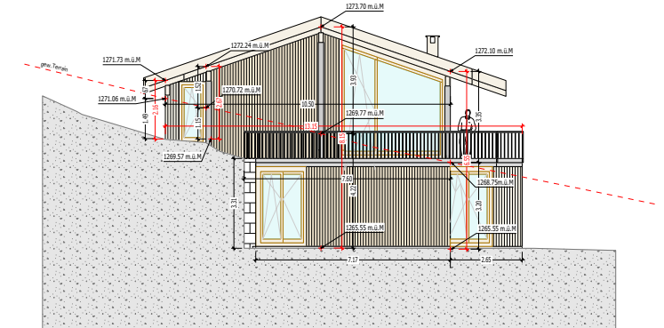
Westfassade
