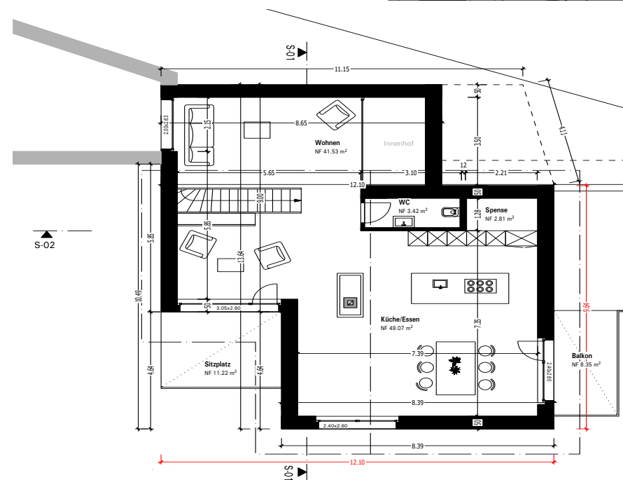
Grundriss Obergeschoss
