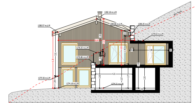
Ostseite
