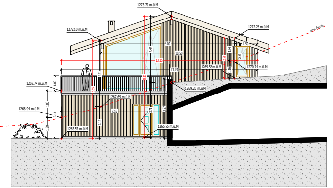
Ostfassade
