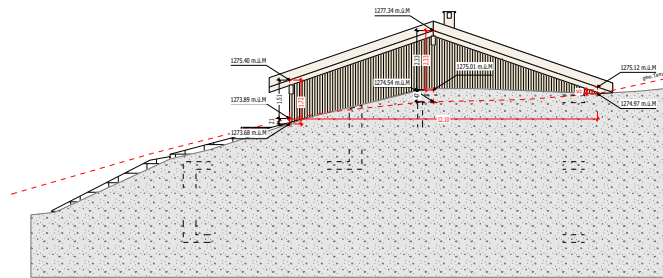
Nordseite
