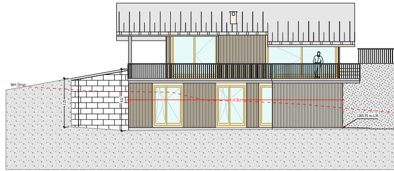
Südfassade
