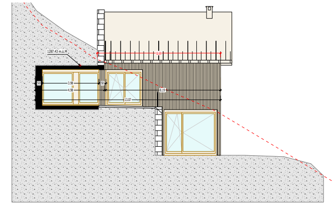
Westfassade
