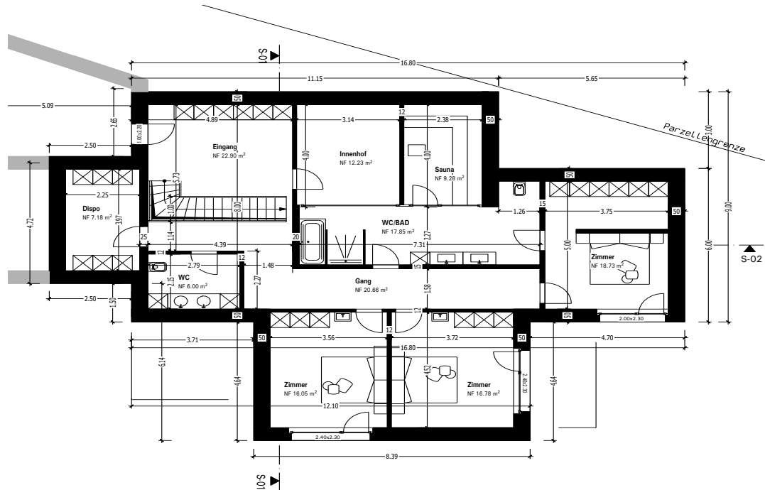
Grundriss Erdgeschoss
