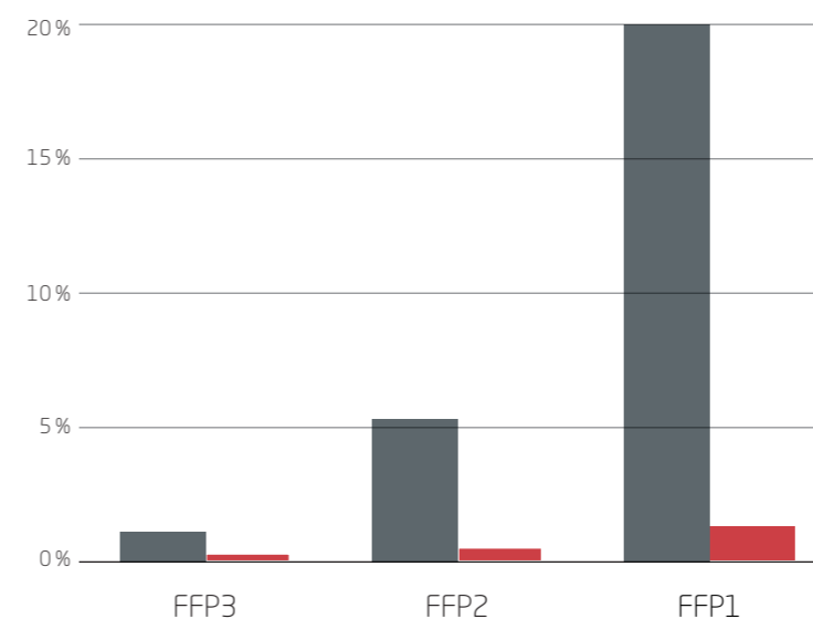
Capacité de filtration Perméabilité aux particules
